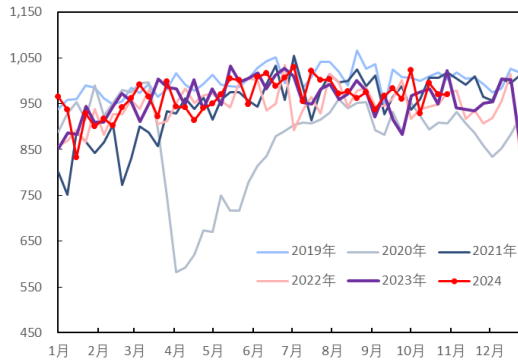
图 65: 美国成品车用汽油产量 (万桶/天)
