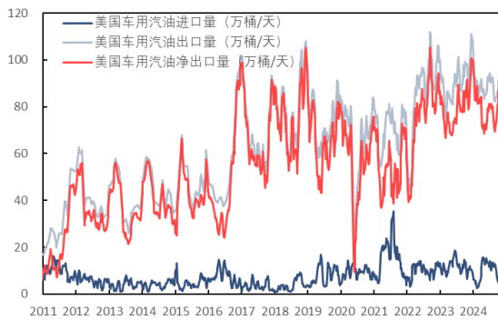
图 72：美国车用汽油进出口情况（万桶/天）
