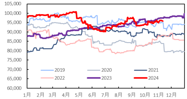
图 13: 350 英尺+自升式钻井平台平均日费 (美元/天)
