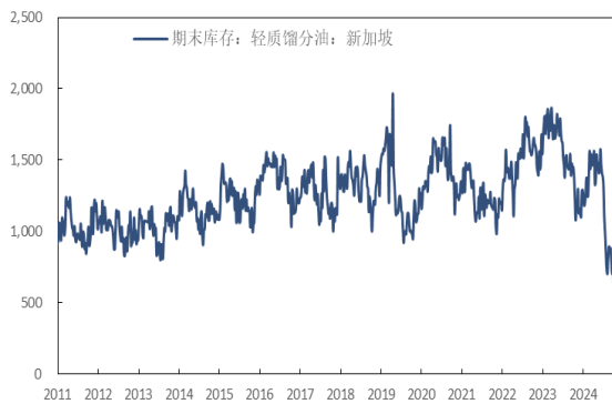
图 86: 新加坡汽油库存 (万桶)
