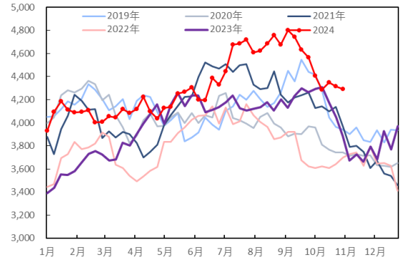
图 85: 美国航空煤油库存 (万桶)
