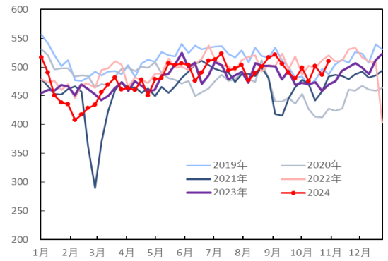
图 66: 美国柴油产量 (万桶/天)
