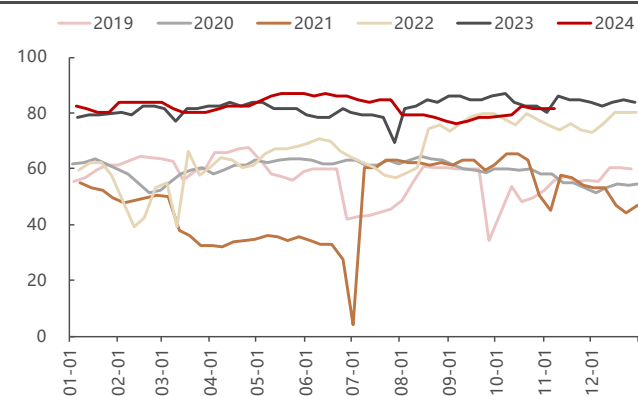
图1：唐山高炉开工率环周持平（%）
