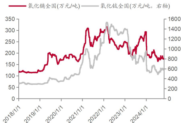
图表 41: 氧化镨&氧化铽价格走势 (万元/吨)
