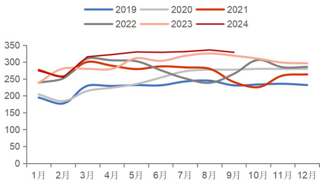
图表 52: 不锈钢月度产量 (万吨)
