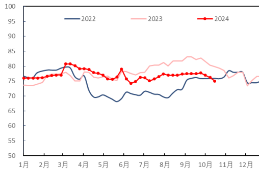
图 32: 中国主营炼厂开工率 (%)
