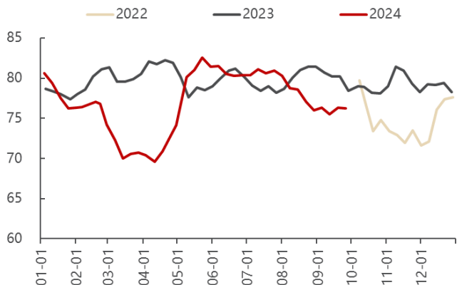
图3：独立焦化企业(100 家)产能利用率下降 (%)
