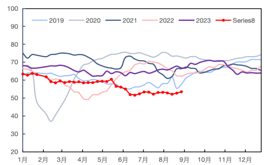
图 33: 山东地炼开工率 (%)
