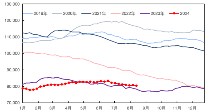
图 39: 美国原油总库存 (万桶)
