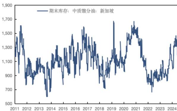
图 84: 新加坡柴油库存 (万桶)
