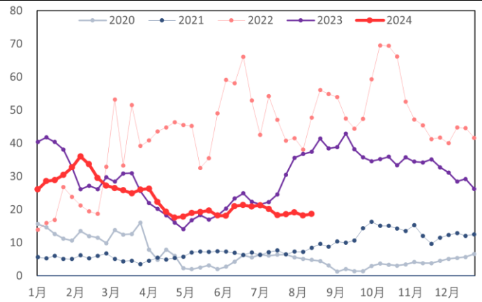
图 26: 原油、欧洲柴油价差 (美元/桶, 美元/桶)
