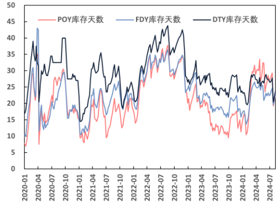
图 65: 聚酯企业的涤纶长丝库存天数 (天)
