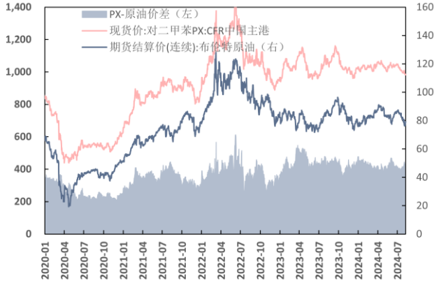
图 51: 原油、PX 价格及价差 (美元/吨, 美元/桶)
