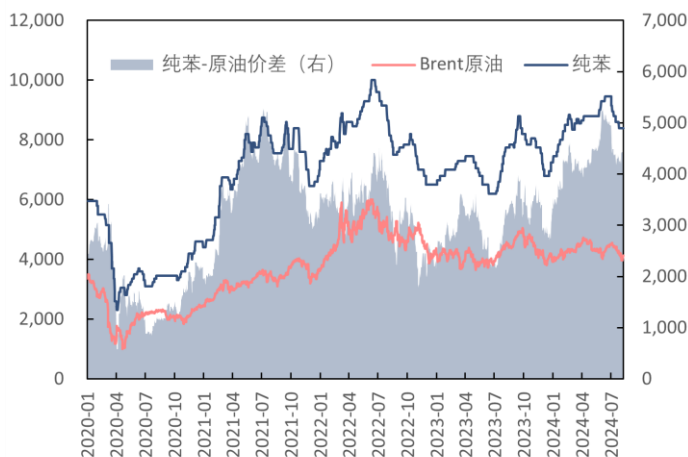
图 35: 原油、纯苯价格及价差 (元/吨, 元/吨)
