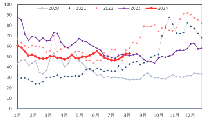
图 8: 原油、国内航煤价差 (美元/桶, 美元/桶)
