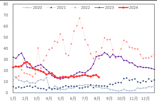
图 10: 原油、新加坡 FOB 柴油价差 (美元/桶, 美元/桶)
