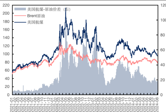
图 54: 原油、美国航煤价格及价差 (美元/桶, 美元/桶)
